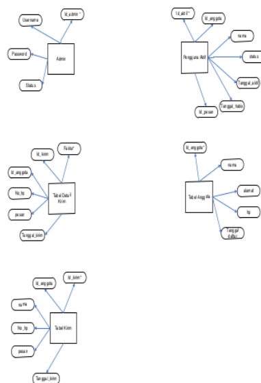
Gambar 5 ERD
