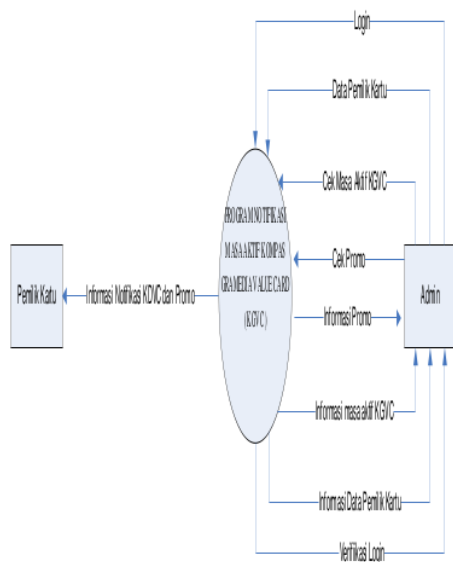
Gambar 3 DFD Konteks
